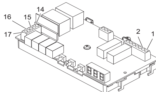
Rysunek: Płytką drukowaną. Patrz też strona 171.
