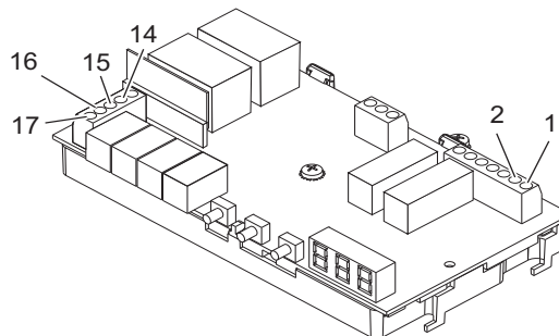
Figura: Placa de mando con circuito impreso. Ver también página 171.
