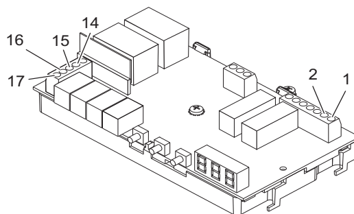
Figure : platine de commande. Voir aussi la page 171.
