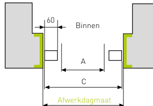
Inbouw tussen de dagopening
