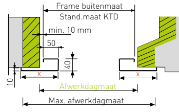
Inbouw voor de dagopening
