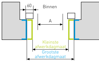
Inbouw achter de dagopening
